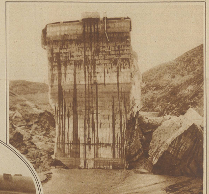
Zur Dammbruch-Katastrophe in Santa Paula (Kalifornien), die über 300 Menschenleben kostete und für viele Millionen Franken Sachwerte vernichtete. Die Ueberreste des geborstenen Damms an der Bruchstelle
