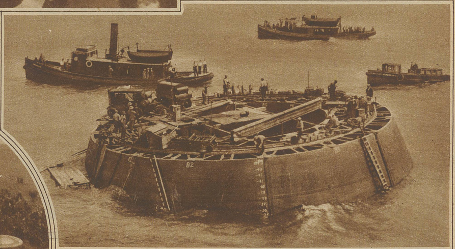
Auf eigenartige Weise muß sich die Stadt Chicago mit Trinkwasser versorgen. Neben den schon bestehenden ließ sie kürzlich eine neue schwimmende Pumpstation im Michigansee verankern, die täglich 700 Millionen Liter aus 50 Meter Tiefe heraufpumpt. Das Bild zeigt die Bauarbeiten an diesem gewaltigen schwimmenden Pumpwerk
