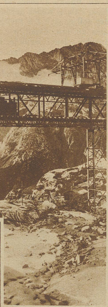
Zum Bau der 380 m langen Gelmersperre, die den Spiegel des Gelmerees um 30 m erhöhen und damit dreizehn Millionen Kubikmeter Stauroum schaffen wird, sind die Geleise der Materialtransportbahn auf die Eisengerüste gelegt worden, die mit einbetoniert werden
