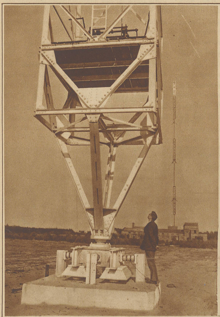
Der größte Rundfunksender Europas ist dieser Tage in Zeesen (Deutschland) eröffnet worden. Unser Bild zeigt das untere Ende eines der beiden 25 m hohen Masten, die nur auf einer kleinen Stahlkugel von 9 cm Durchmesser ruhen
