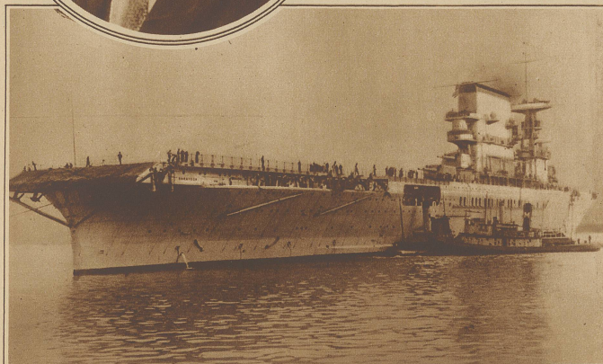
«Saratoga», das größte Flugzeug-Mutterschiff, ist vor kurzem von der amerikanischen Marine in Dienst genommen worden. Es hat eine Wasserverdrängung von 35 000 Tonnen und eine Länge von gegen 300 m. Im Innern des Schiffes haben 120 flugbereite Aeroplane Platz, die binnen wenigen Minuten auf Deck gehoben und gestartet werden können
