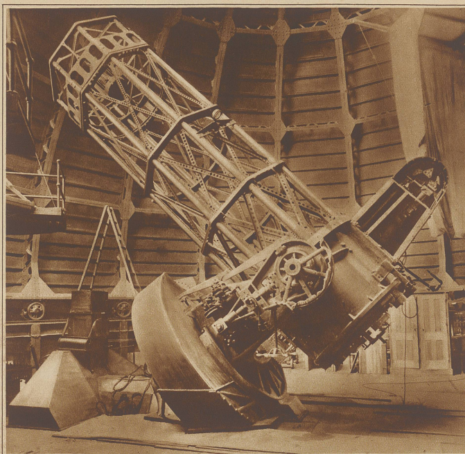
Spiegelteleskop der Mt. Wilson-Sternwarte in Kalifornien. Die Oeffnung beträgt 180 cm. Der Aufsatz rechts ist ein großer Spektrograph zur genauen Untersuchung des Sternlichtes
