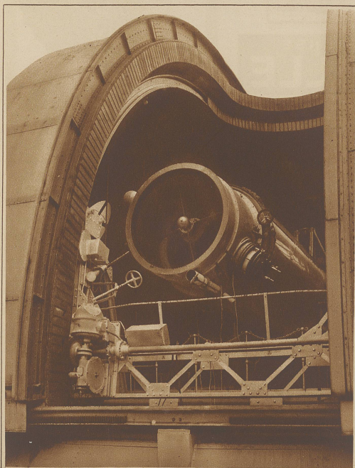
Das vordere Ende des Spiegelteleskops der Sternwarte Berlin-Babelsberg Im Rohrinne ist der schief gestellte Planspiegel sichtbar, der das vom Hauptspiegel kommende Licht in die Kassetteneinrichtung rechts wirft
