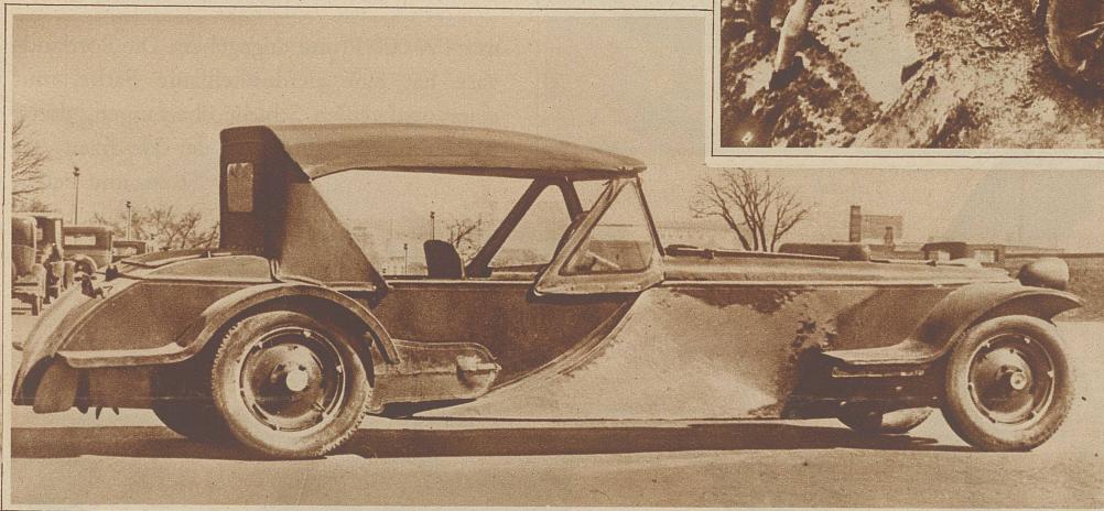
Das neue Amphibienauto des amerikanischen Erfinders Daubenberg, das sich ebensogut auf dem Lande wie im Wasser vorwärtsbewegen kann. Der Antrieb der Hinterräder kann im Wasser durch eine einfache Umschaltung auf eine Schiffsschraube übertragen werden
