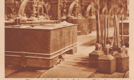
Wagen mit frischer Tonerde. Rechts neue Elektroden
