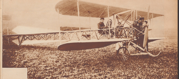
Die dritte Flugzeug der Brüder Dufaux war der 1909 gebaute Kampfdoppeldecker von 275 m Spannweite, 850 m Länge, 14 Quadratmeter Tragfläche und 210 kg Gewicht. Mit diesem ersten schweizerischen Flugzeug erzielten Armand und Henri Dufaux, sowie die Schweizerpiloten Tullio, Fallois und Thirion 1911/12 merkbare Erfolge. Es war dies nach der Flugzeug, mit dem im Januar 1911 die ersten Militärflügeversuche in der Schweiz unternommen wurden. Le troisième appareil des frères Dufaux (1909) mesurant 8,5 m de long et portant 210 kilos. C'est par cet appareil que les Dufaux, Tullio, Fallois et Thirion obtinrent, en 1911, les premiers résultats. C'est également sur cet appareil que fut procédé, en 1911, au premier essai d'aviation militaire suisse.
