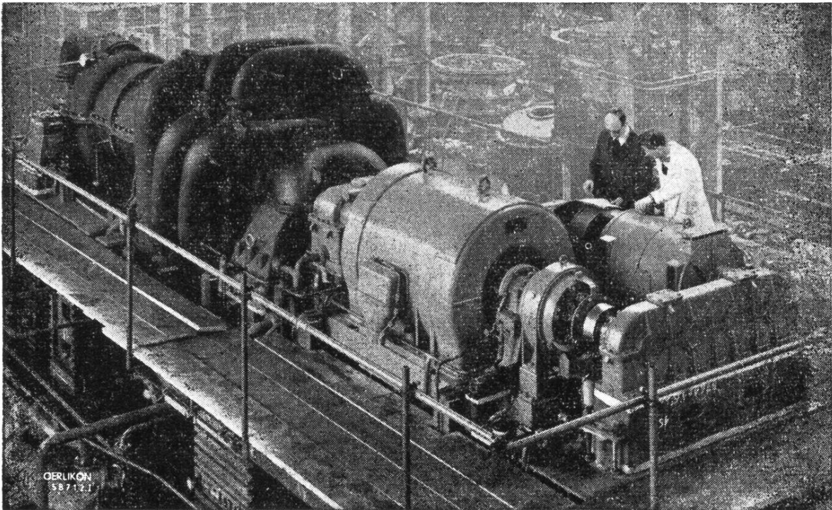
Bild: Gasturbinenanlage auf dem Versuchsstand.
